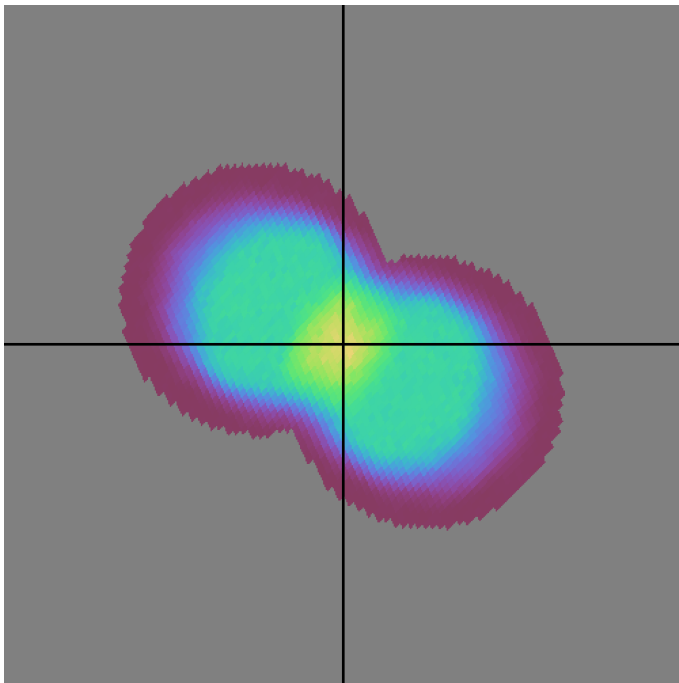
too_10_1v3.4_10yrs g band: DD:EDFS NVisits
