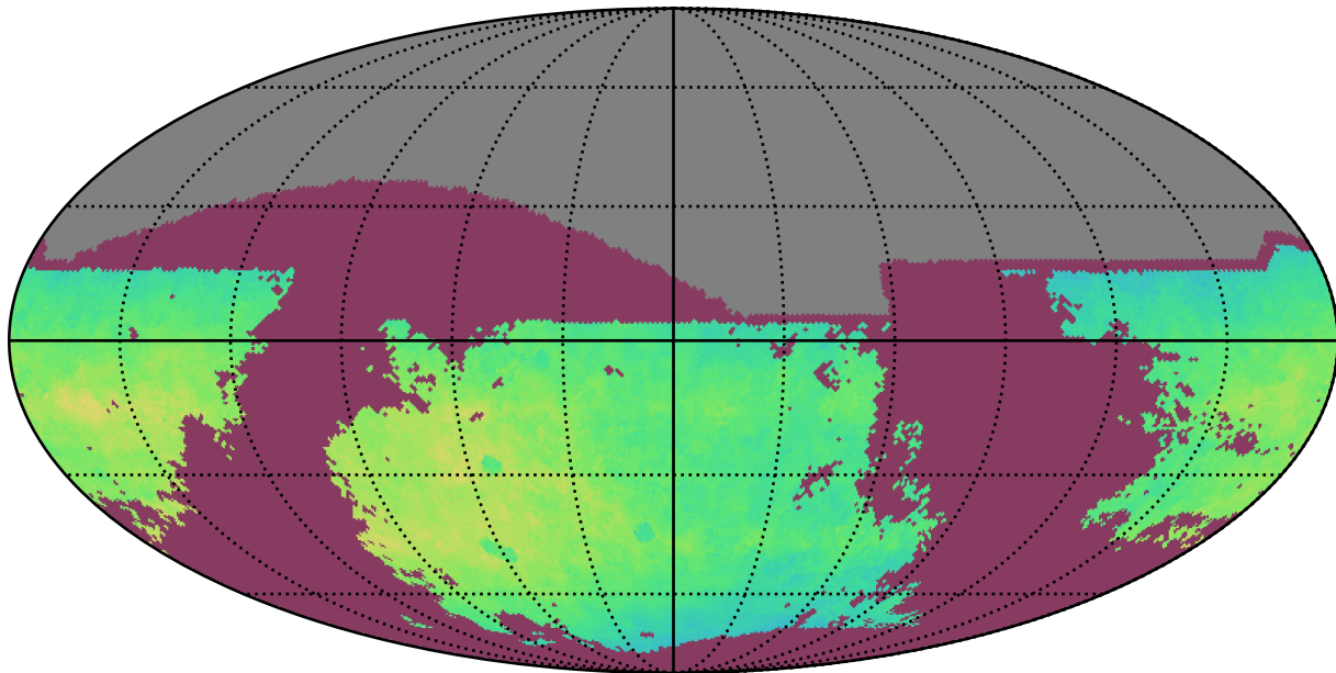
too_100_4v3.4_10yrs i: NgalScale
