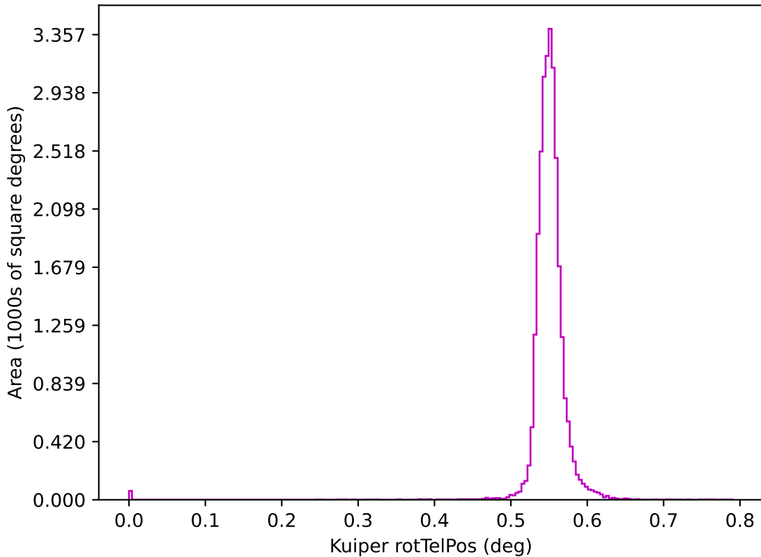
too_100_4v3.4_10yrs z: Kuiper rotTelPos
