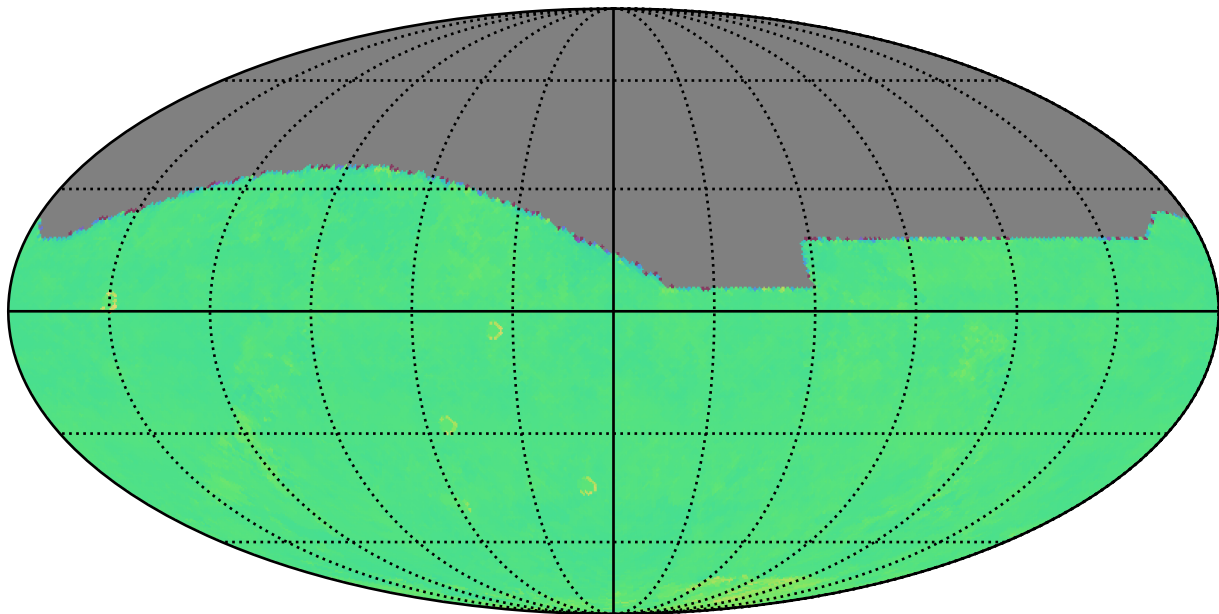
too_100_4v3.4_10yrs r: Kuiper rotTelPos
