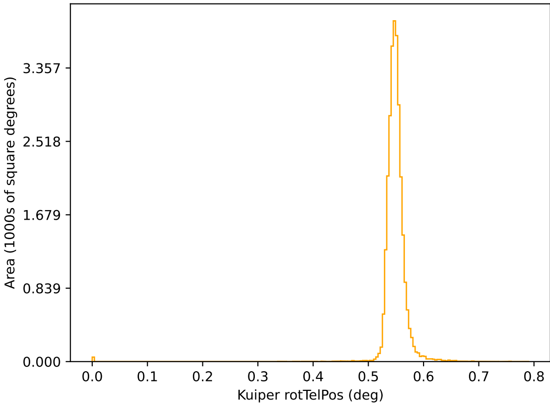
too_100_4v3.4_10yrs r: Kuiper rotTelPos
