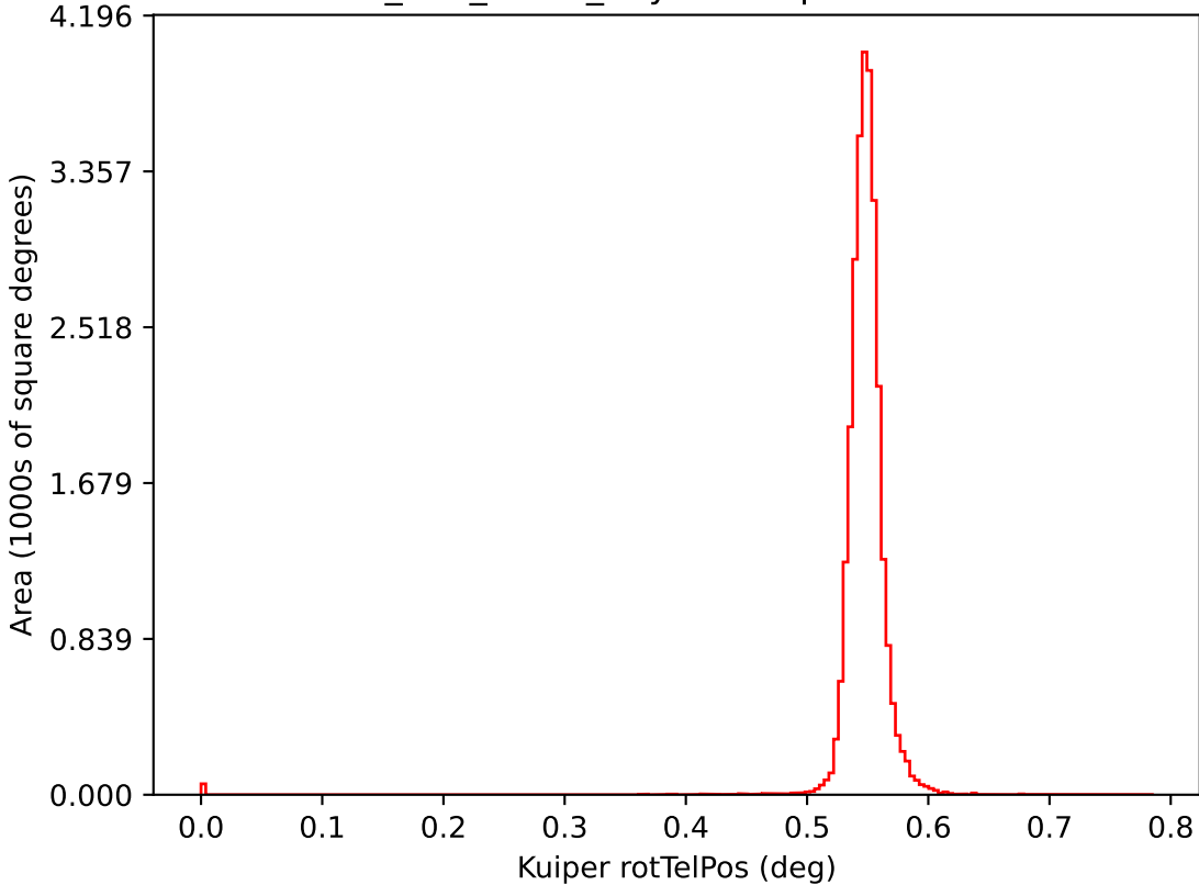
too_100_4v3.4_10yrs i: Kuiper rotTelPos
