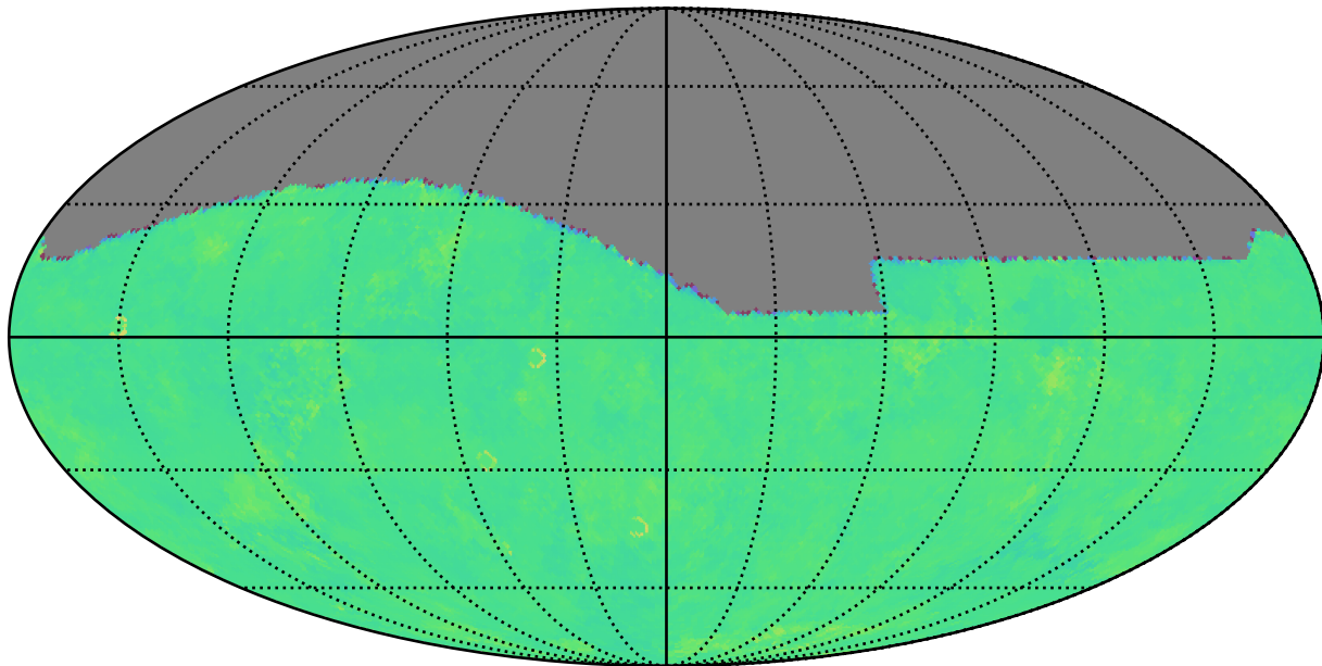
too_100_4v3.4_10yrs g: Kuiper rotTelPos
