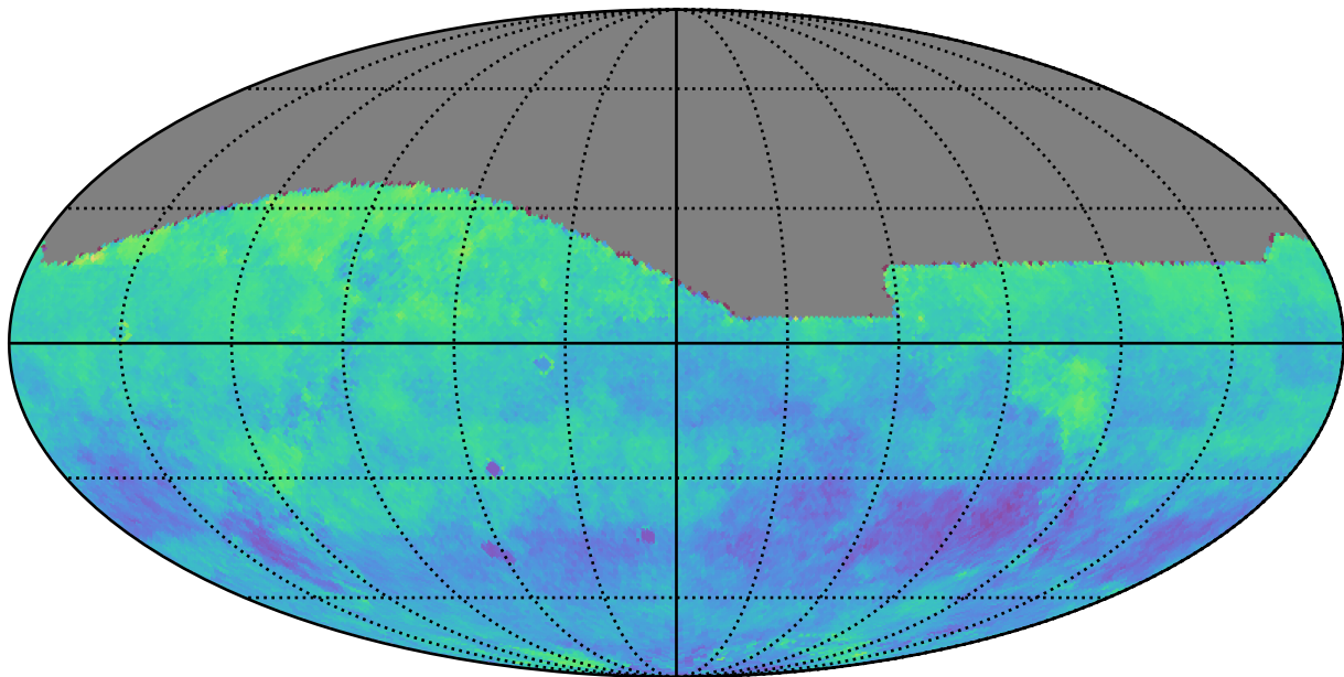
too_100_4v3.4_10yrs z: Kuiper rotSkyPos
