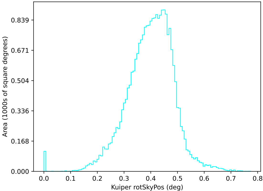
too_100_4v3.4_10yrs u: Kuiper rotSkyPos
