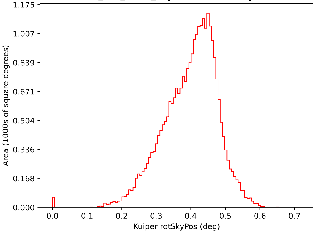
too_100_4v3.4_10yrs i: Kuiper rotSkyPos
