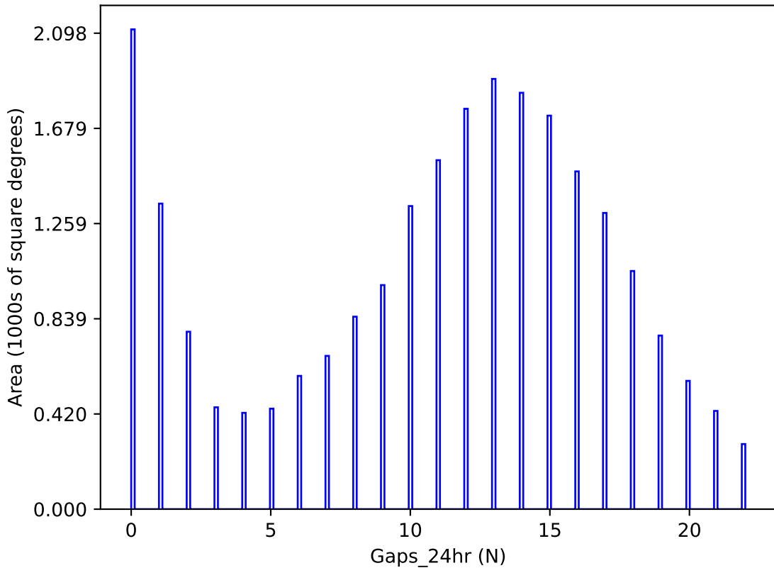
too_100_4v3.4_10yrs y band: Gaps_24hr
