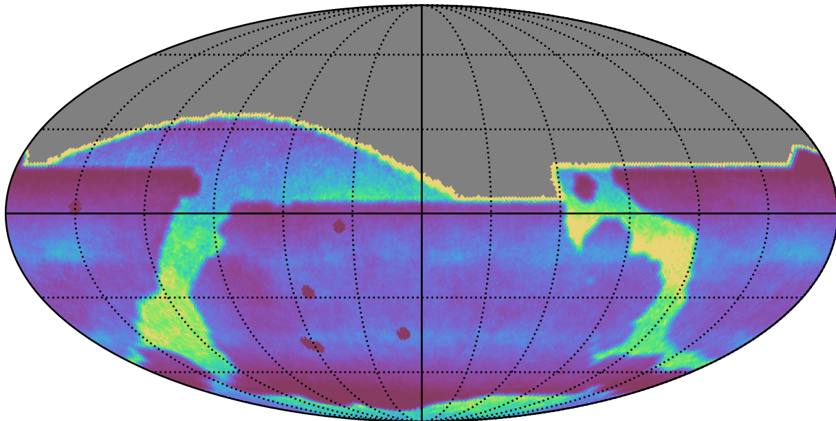
too_100_4v3.4_10yrs : DCRprecision
