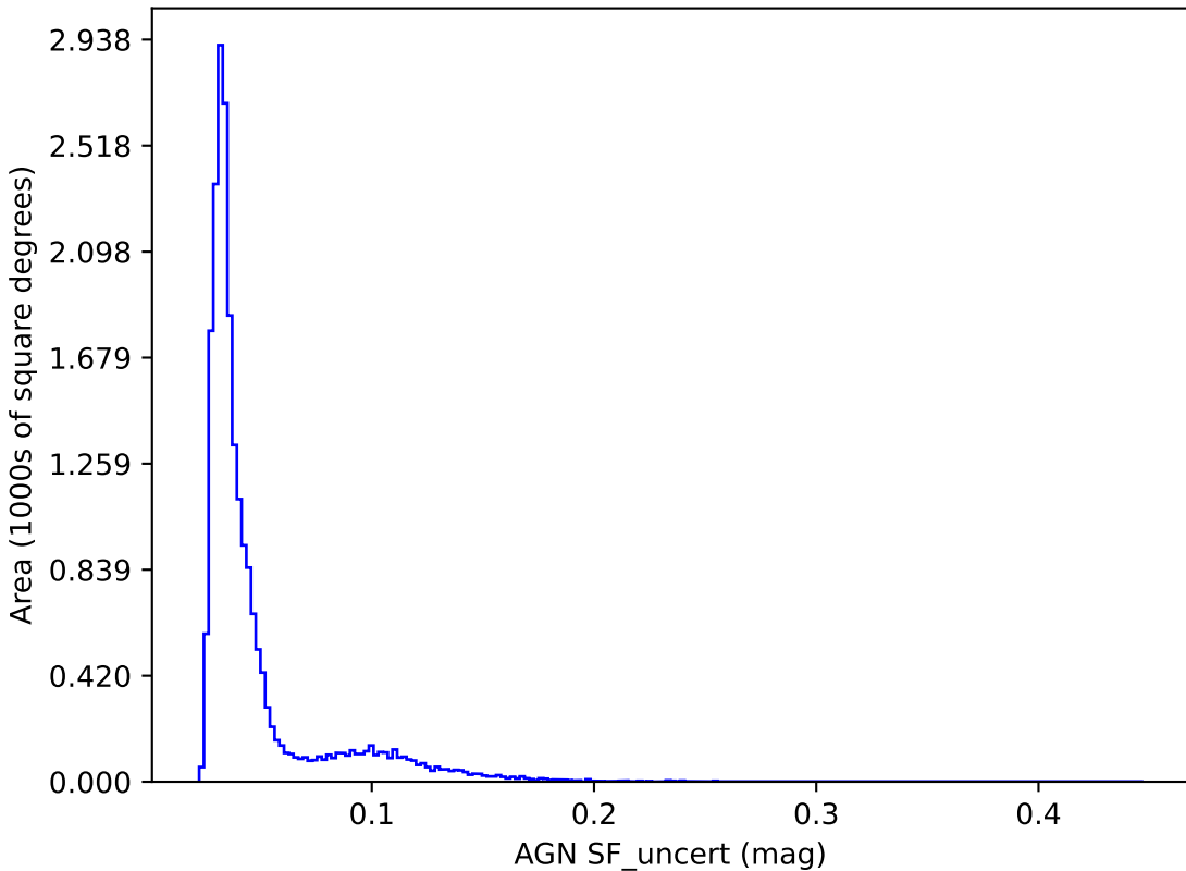
too_100_4v3.4_10yrs y band: AGN SF_uncert
