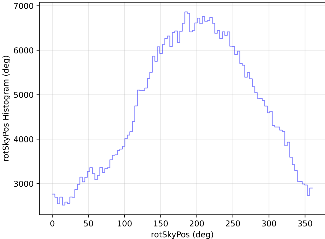
too_100_4v3.4_10yrs WFD r band: rotSkyPos Histogram
