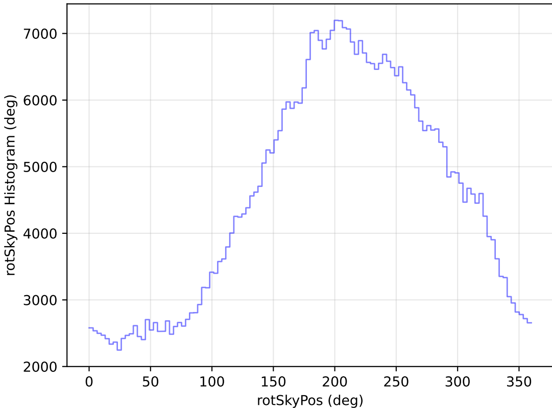
too_100_4v3.4_10yrs WFD i band: rotSkyPos Histogram
