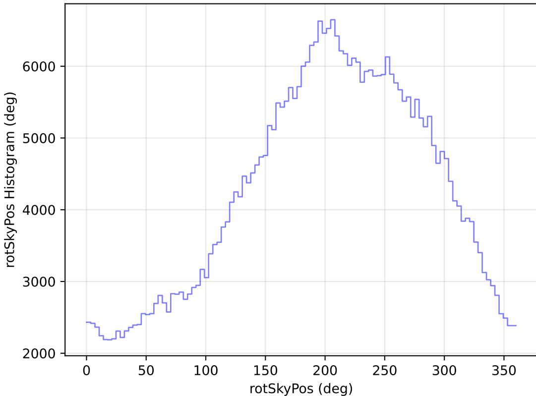
too_100_4v3.4_10yrs All sky z band: rotSkyPos Histogram
