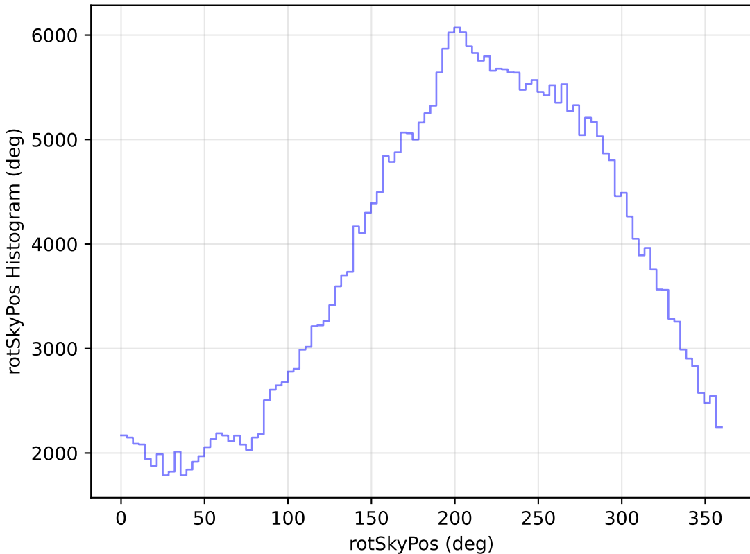
too_100_4v3.4_10yrs All sky y band: rotSkyPos Histogram
