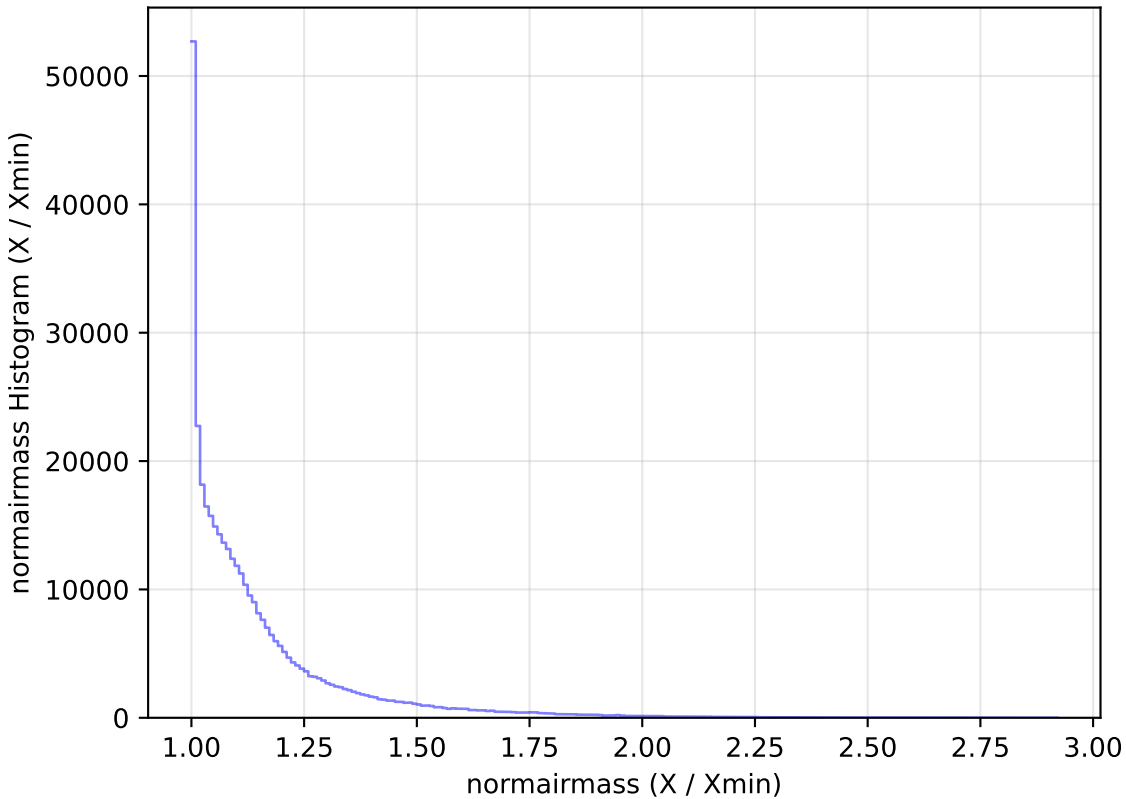
too_100_4v3.4_10yrs WFD y band: normairmass Histogram
