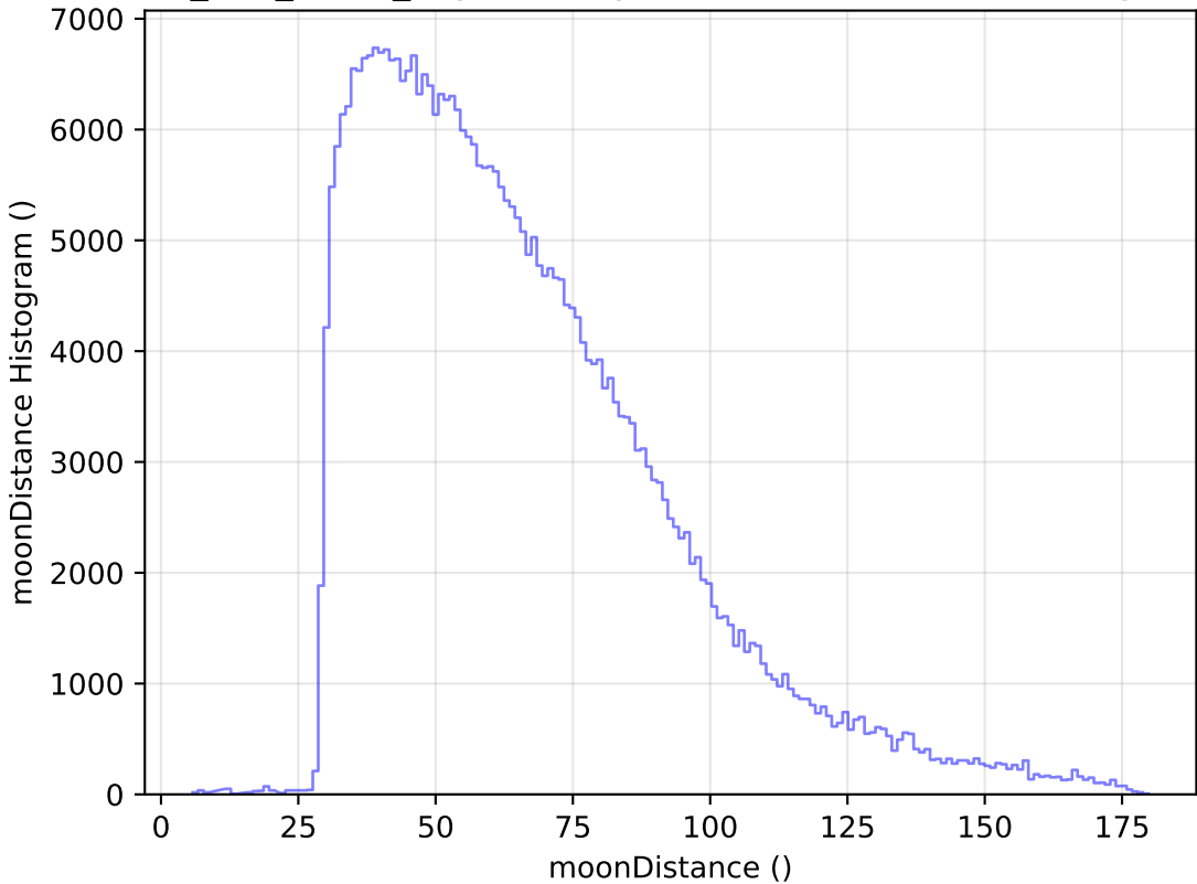
too_100_4v3.4_10yrs WFD y band: moonDistance Histogram
