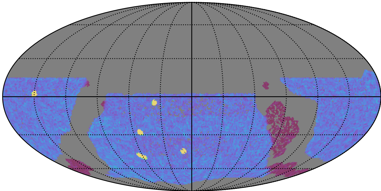
too_100_4v3.4_10yrs WFD y band: NVisits
