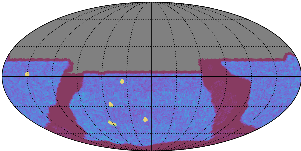
too_100_4v3.4_10yrs All sky y band: NVisits
