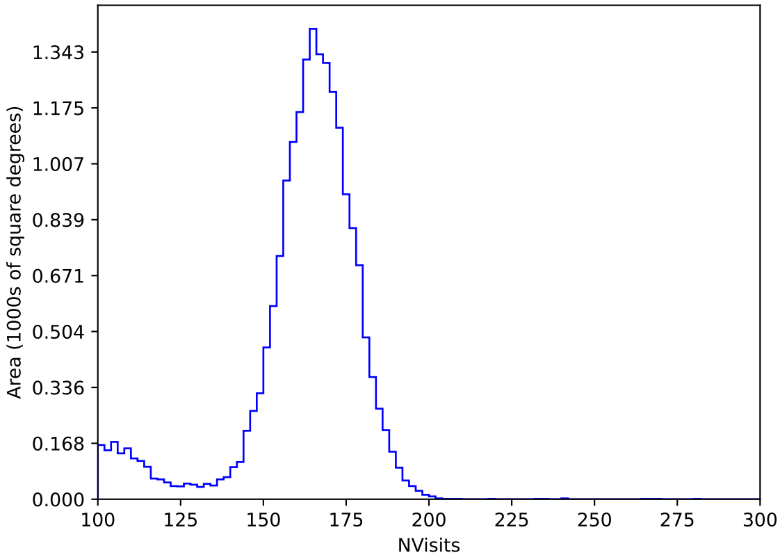
too_100_4v3.4_10yrs All sky y band: NVisits
