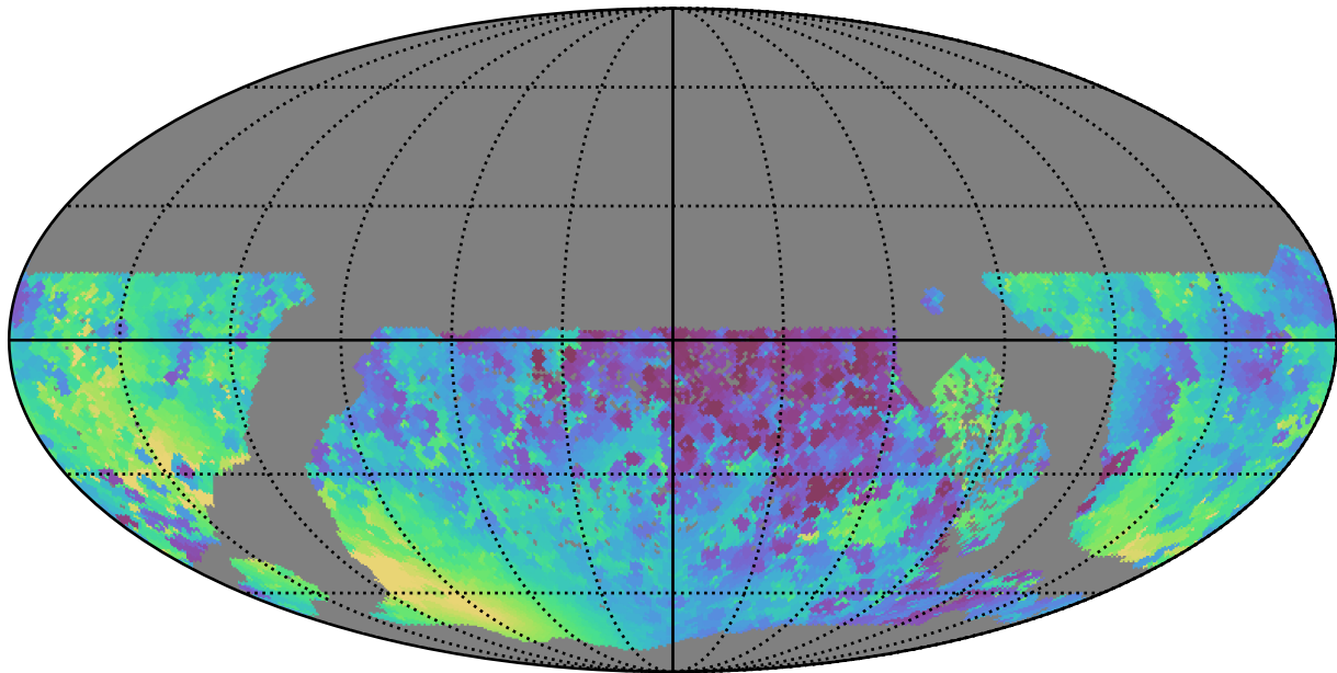
too_100_4v3.4_10yrs WFD y band: Min solarElong
