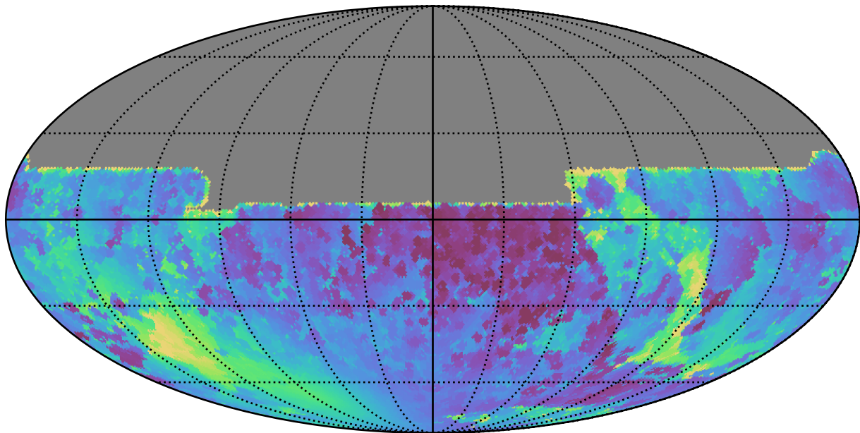
too_100_4v3.4_10yrs All sky y band: Min solarElong
