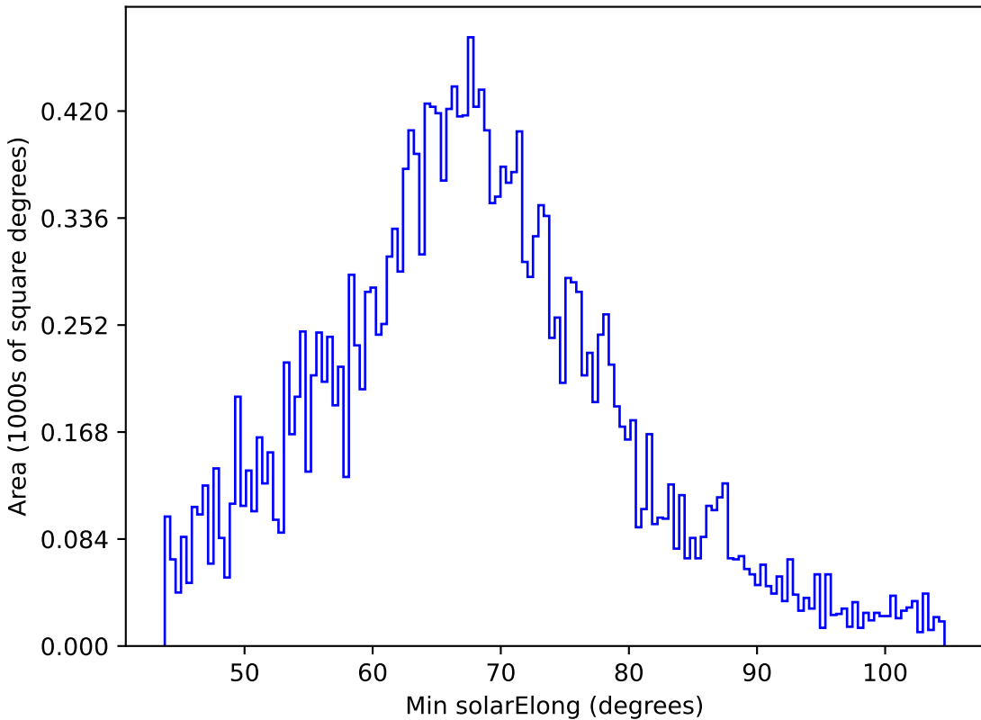
too_100_4v3.4_10yrs All sky y band: Min solarElong
