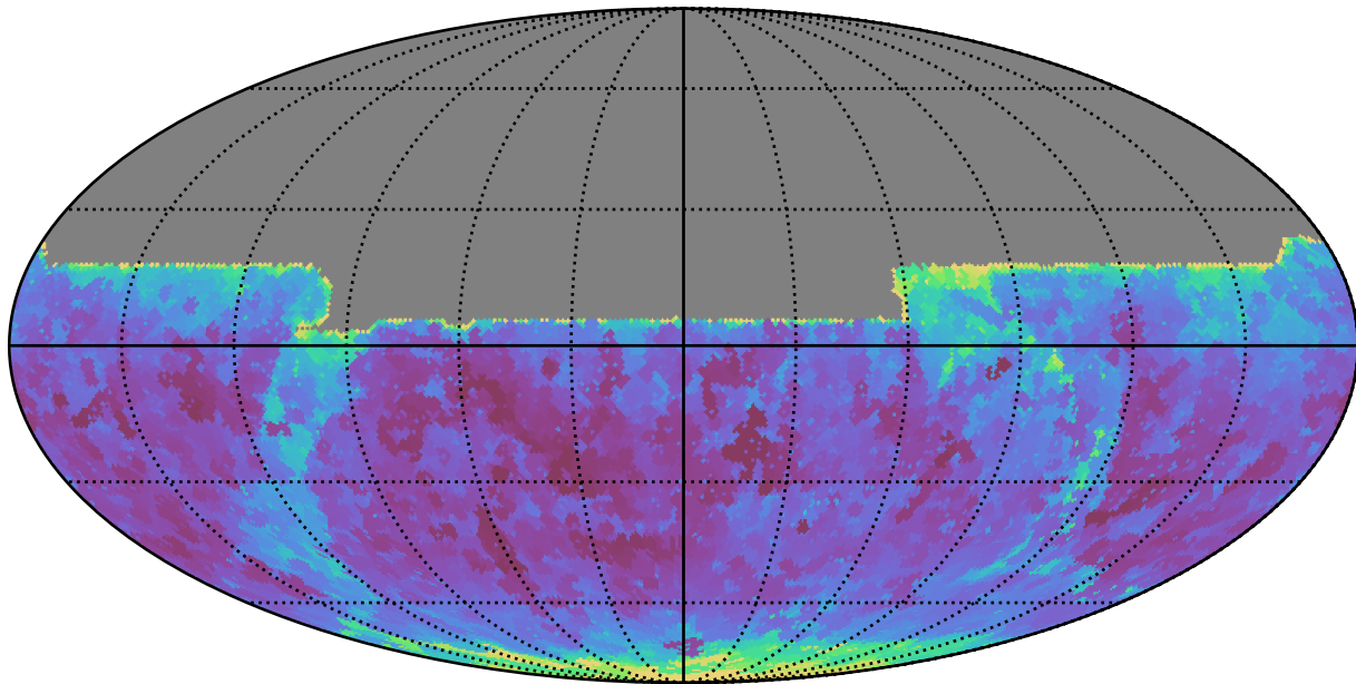
too_100_4v3.4_10yrs All sky y band: Min seeingEff
