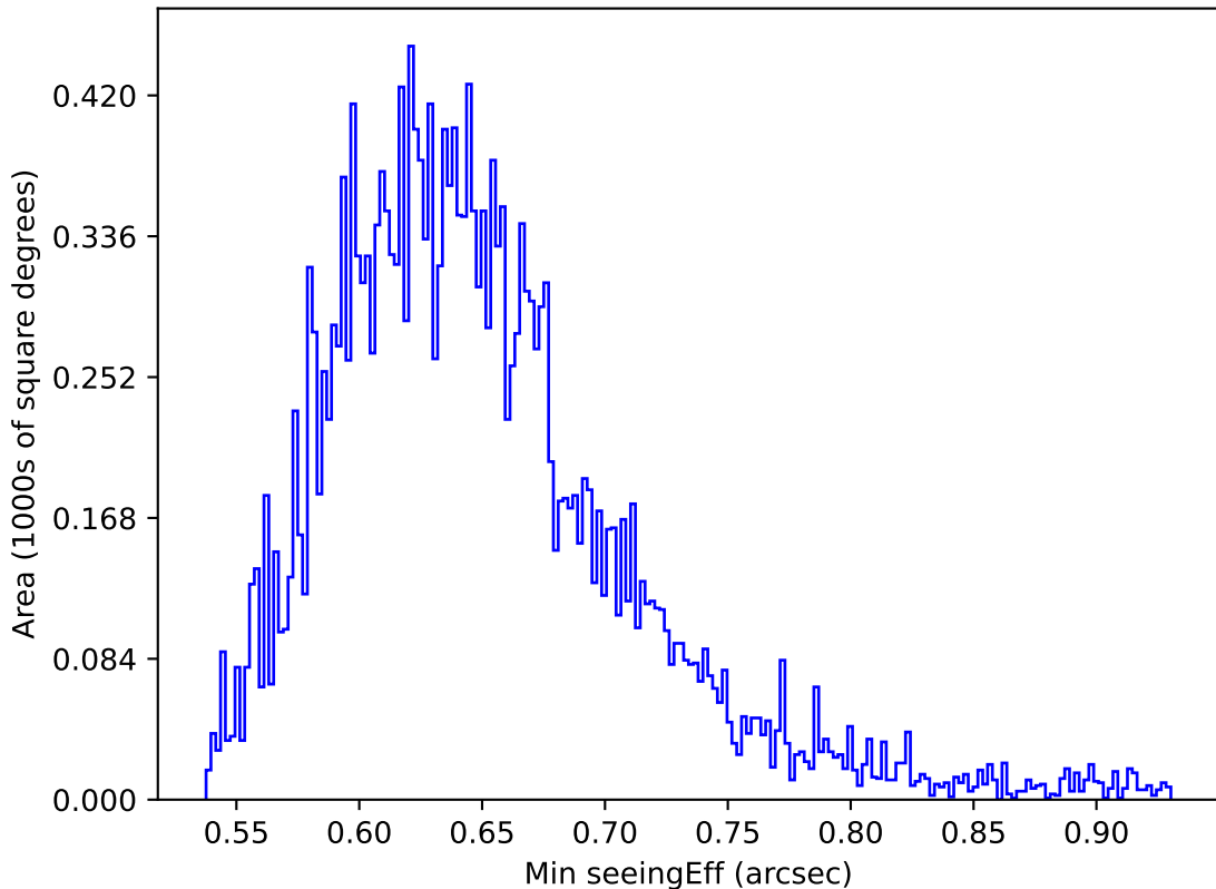
too_100_4v3.4_10yrs All sky y band: Min seeingEff
