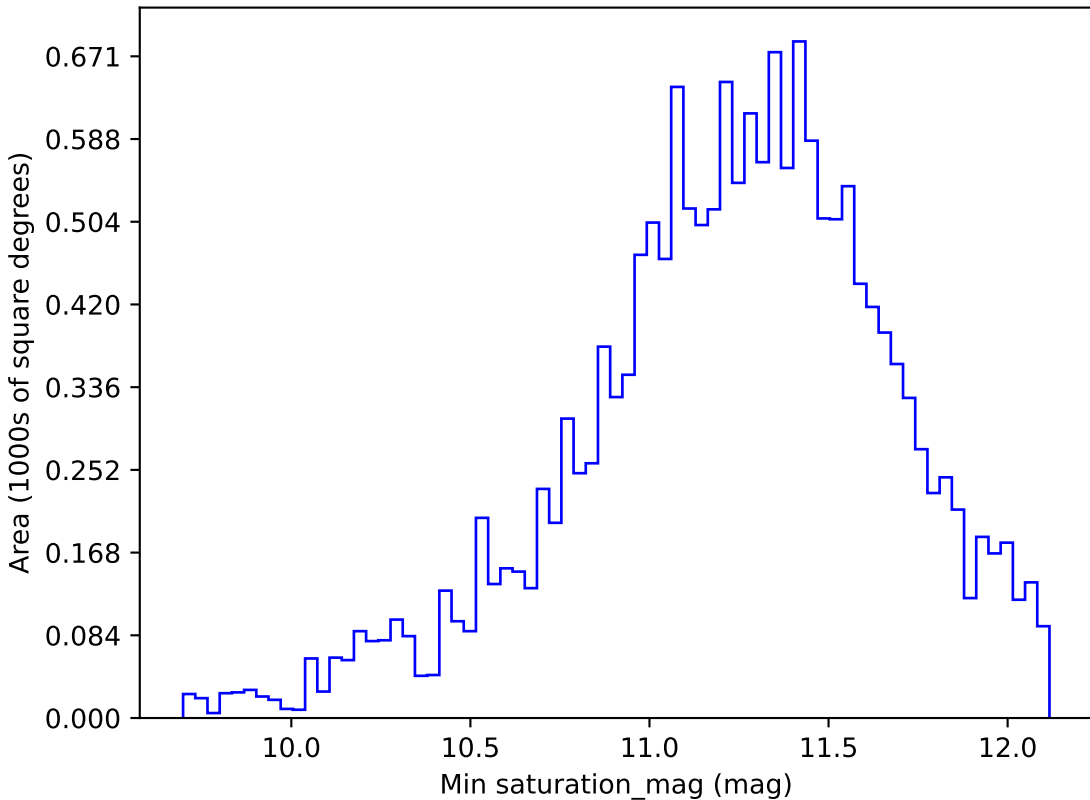
too_100_4v3.4_10yrs WFD y band: Min saturation_mag
