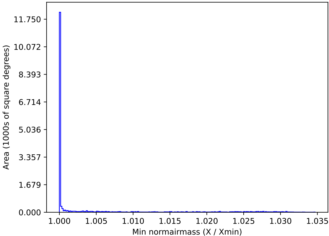
too_100_4v3.4_10yrs WFD z band: Min normairmass
