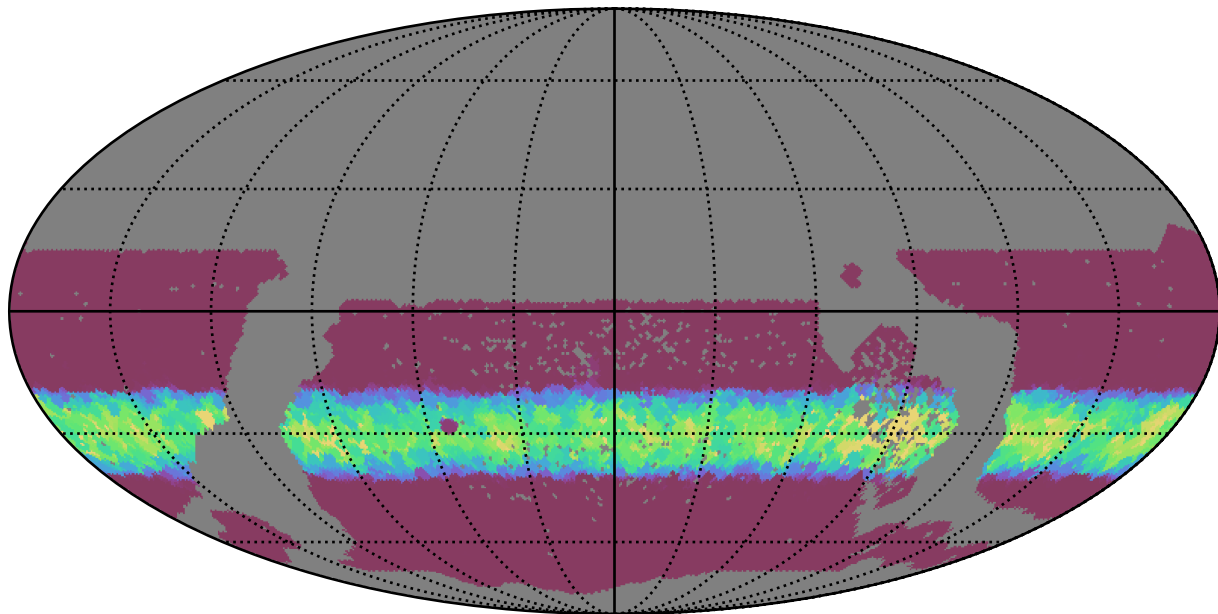
too_100_4v3.4_10yrs WFD y band: Min normairmass
