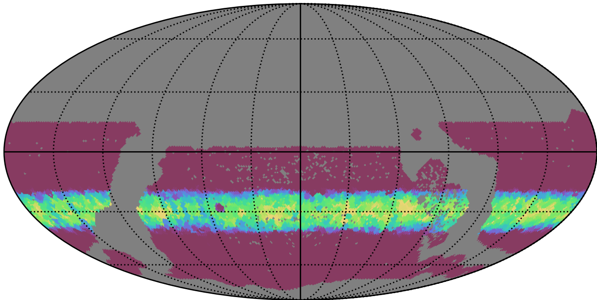
too_100_4v3.4_10yrs WFD i band: Min normairmass
