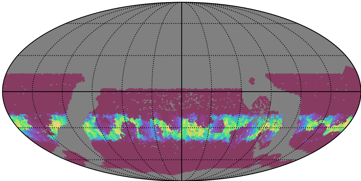
too_100_4v3.4_10yrs WFD g band: Min normairmass
