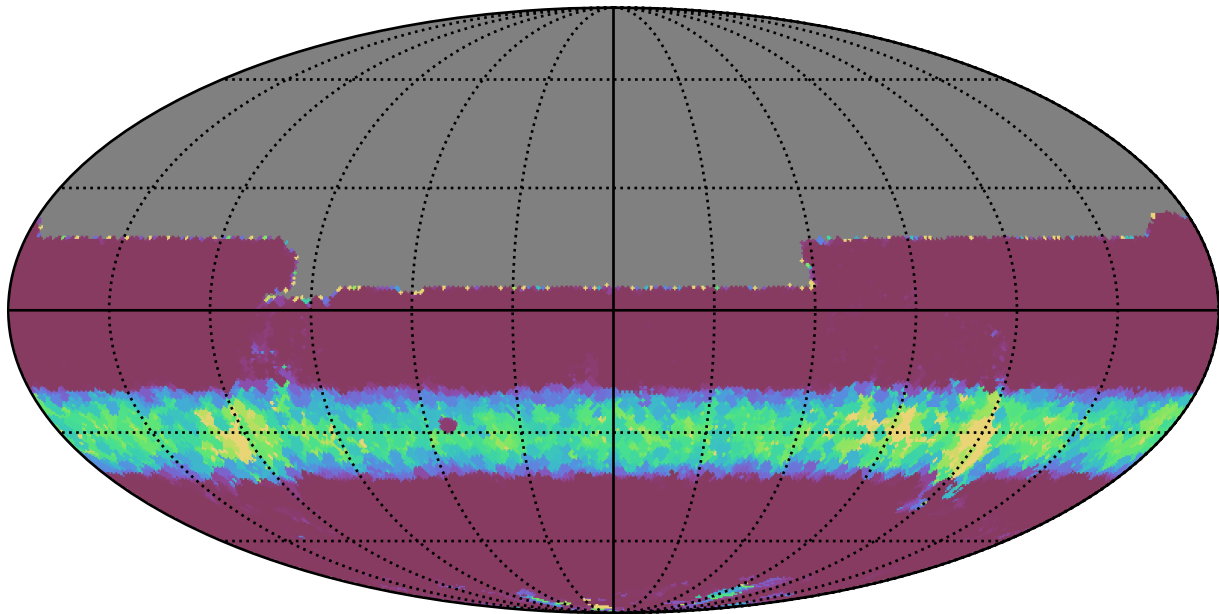
too_100_4v3.4_10yrs All sky y band: Min normairmass
