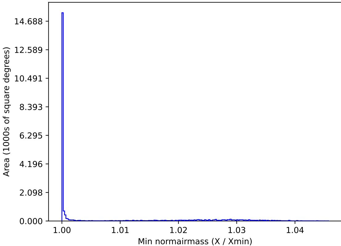
too_100_4v3.4_10yrs All sky y band: Min normairmass
