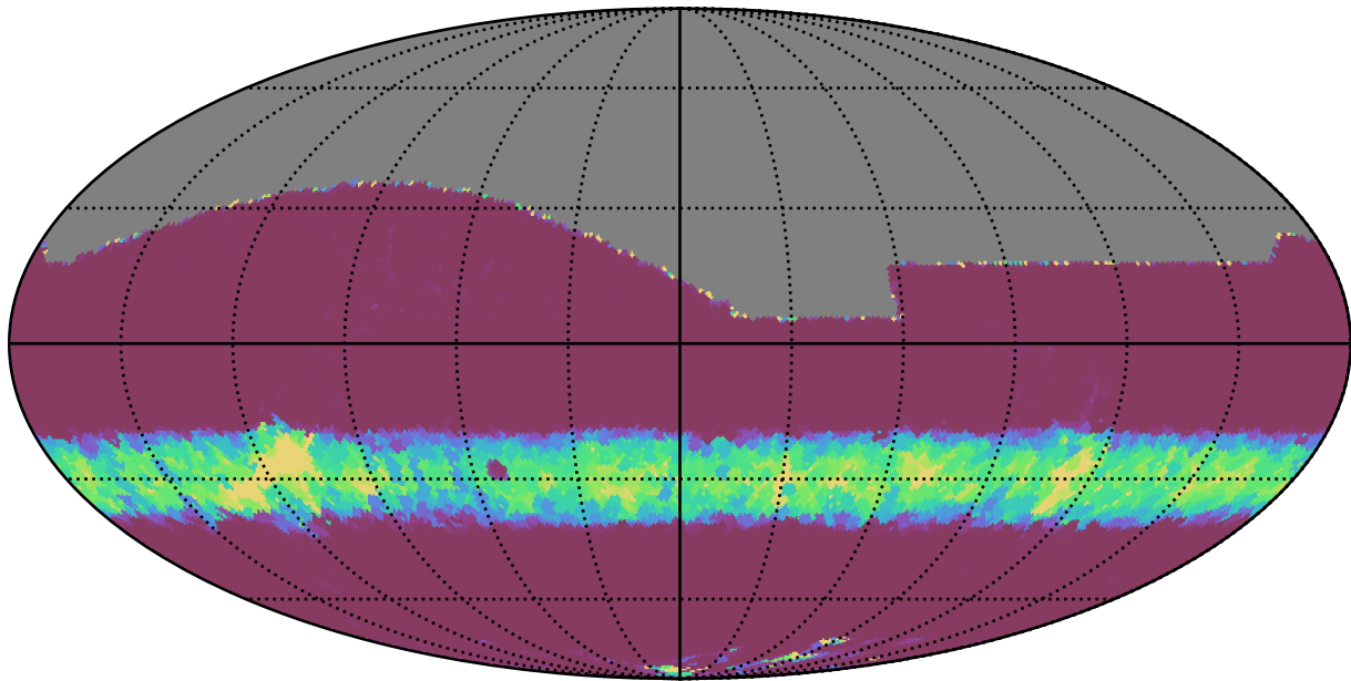
too_100_4v3.4_10yrs All sky i band: Min normairmass
