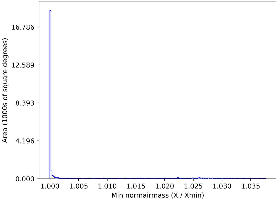
too_100_4v3.4_10yrs All sky i band: Min normairmass
