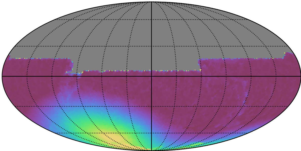
too_100_4v3.4_10yrs All sky y band: Min moonDistance
