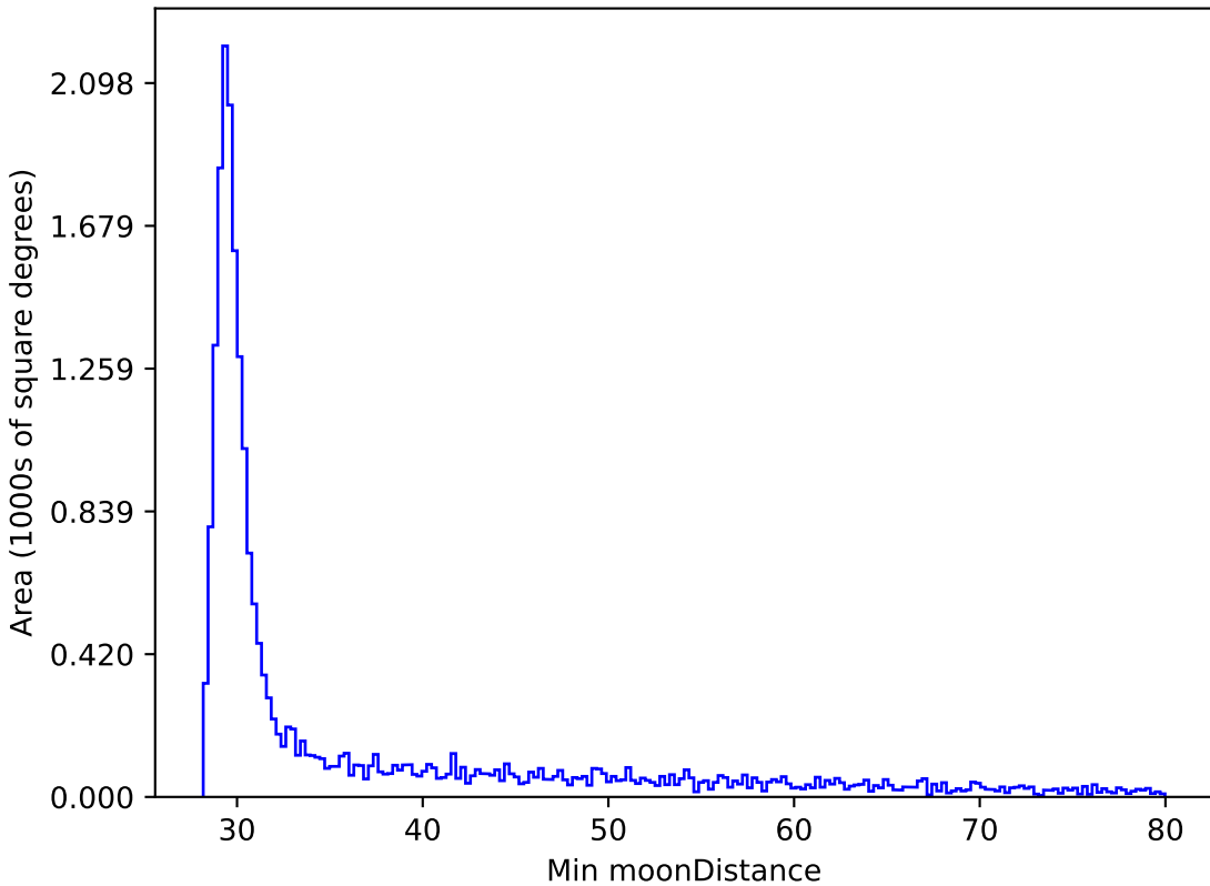
too_100_4v3.4_10yrs All sky y band: Min moonDistance
