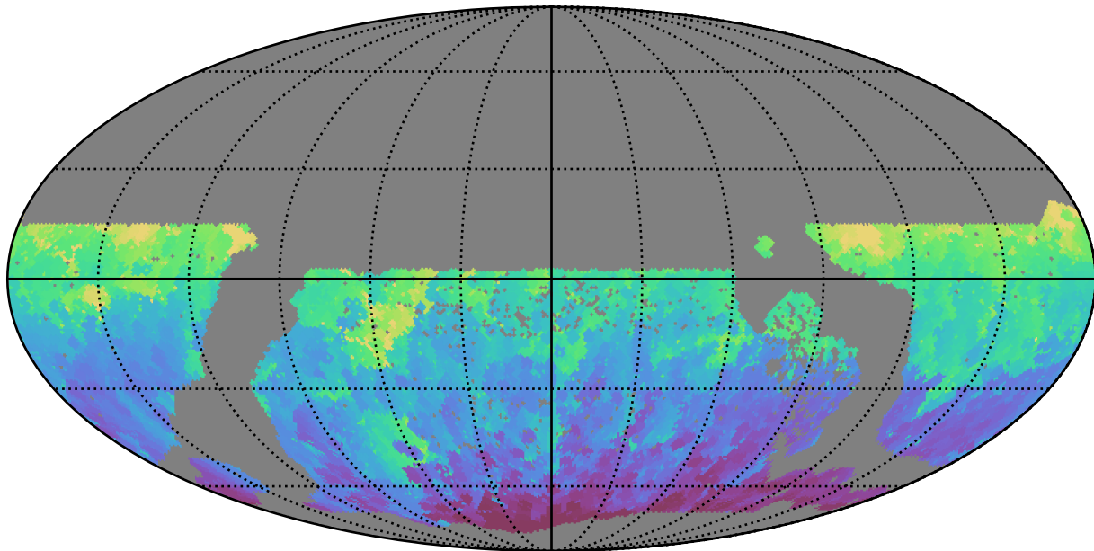
too_100_4v3.4_10yrs WFD z band: Min HA
