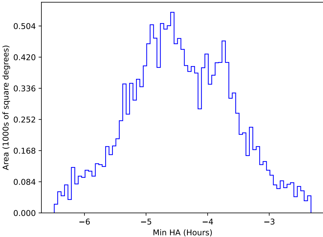
too_100_4v3.4_10yrs WFD z band: Min HA
