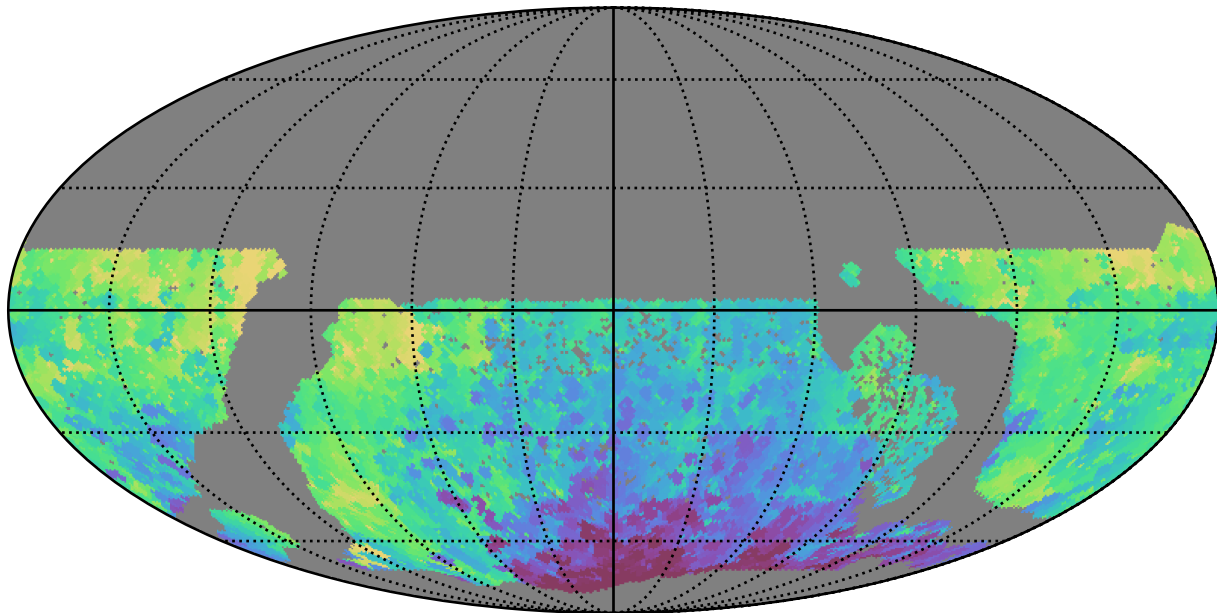
too_100_4v3.4_10yrs WFD y band: Min HA
