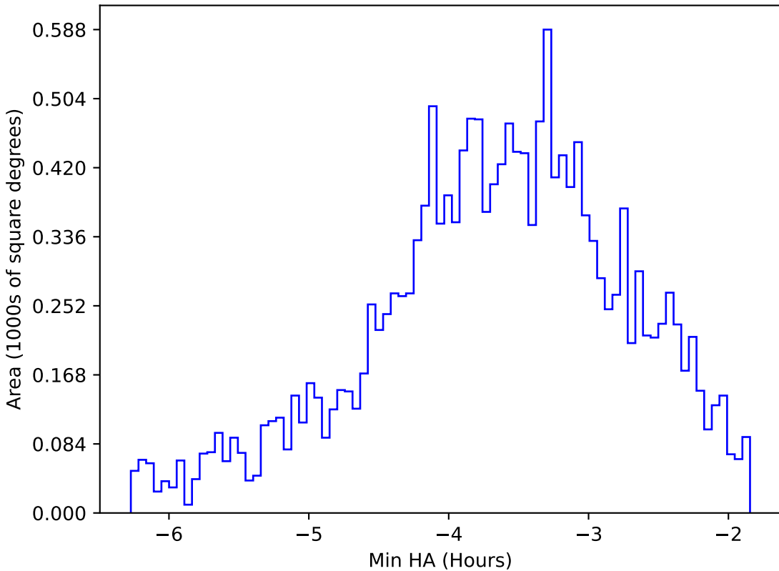
too_100_4v3.4_10yrs WFD y band: Min HA
