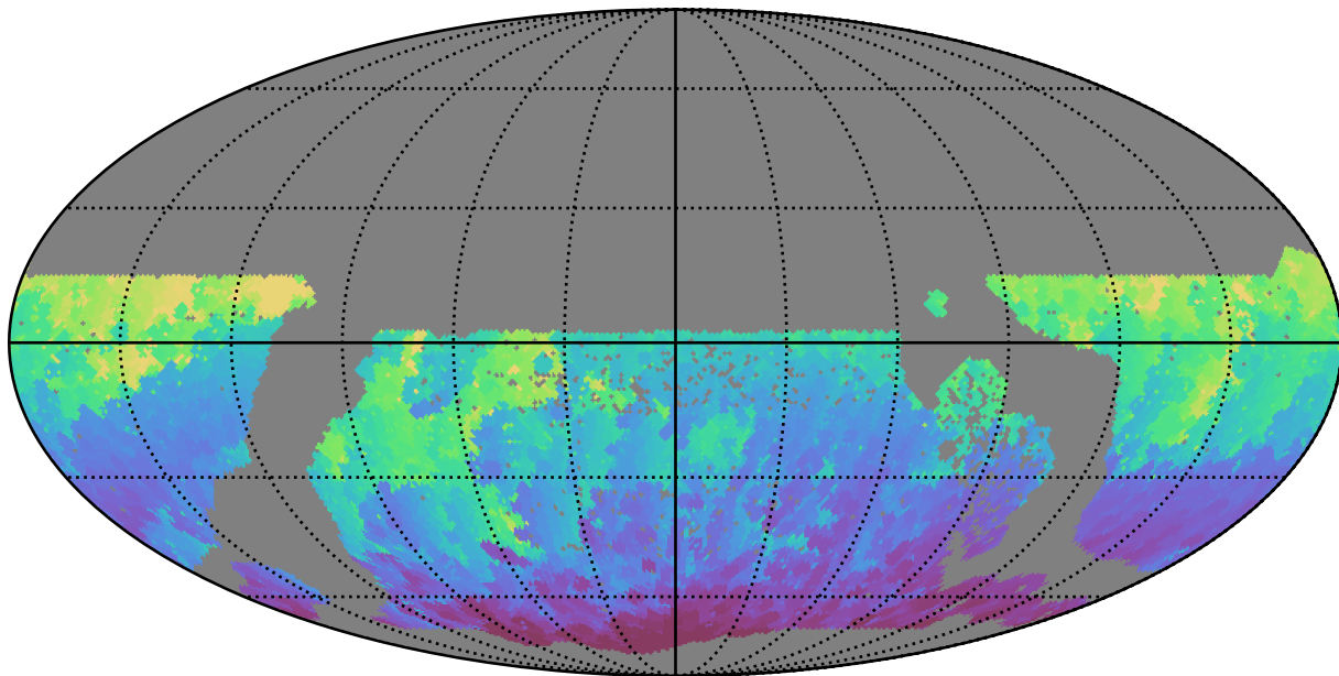
too_100_4v3.4_10yrs WFD i band: Min HA
