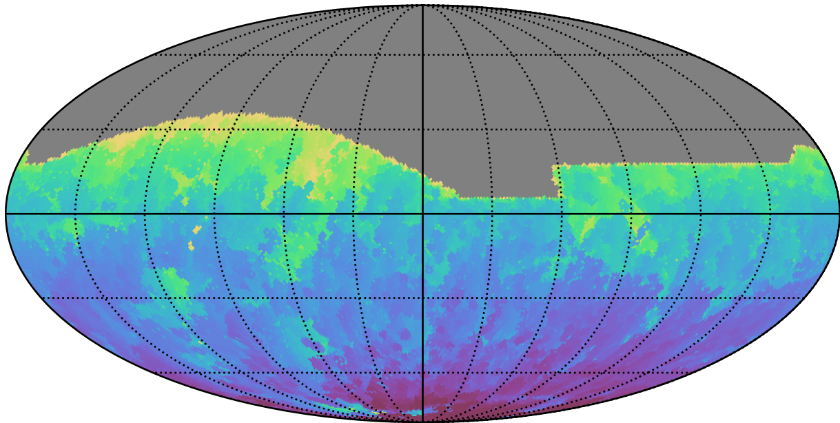
too_100_4v3.4_10yrs All sky z band: Min HA
