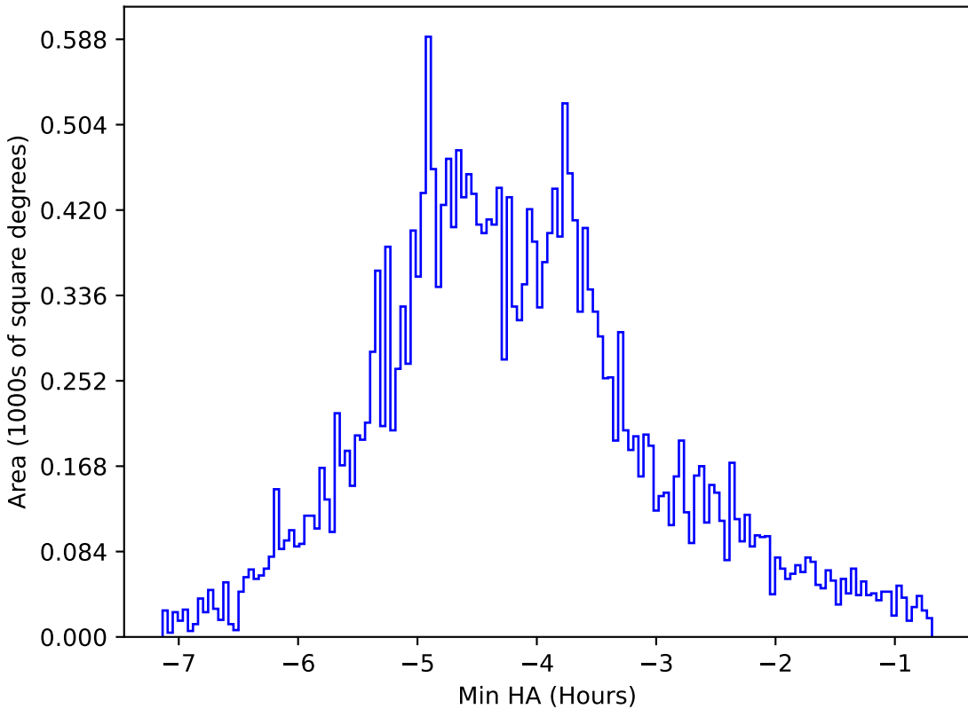
too_100_4v3.4_10yrs All sky z band: Min HA
