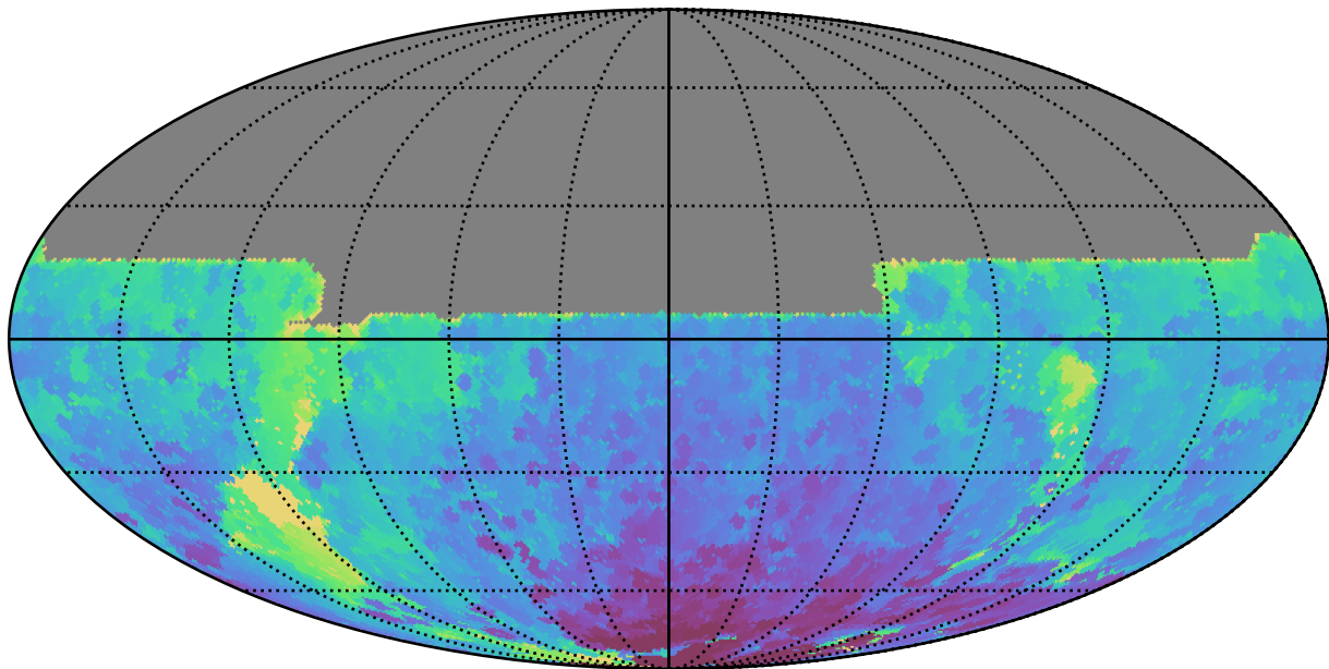
too_100_4v3.4_10yrs All sky y band: Min HA
