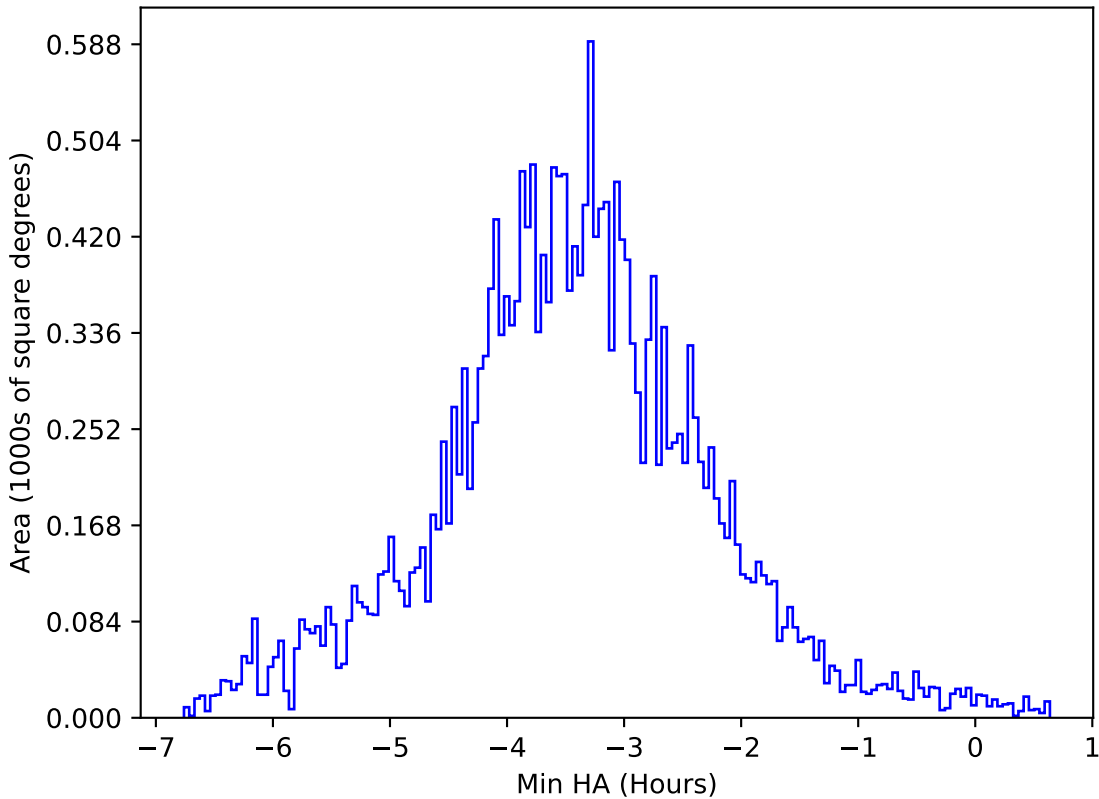
too_100_4v3.4_10yrs All sky y band: Min HA
