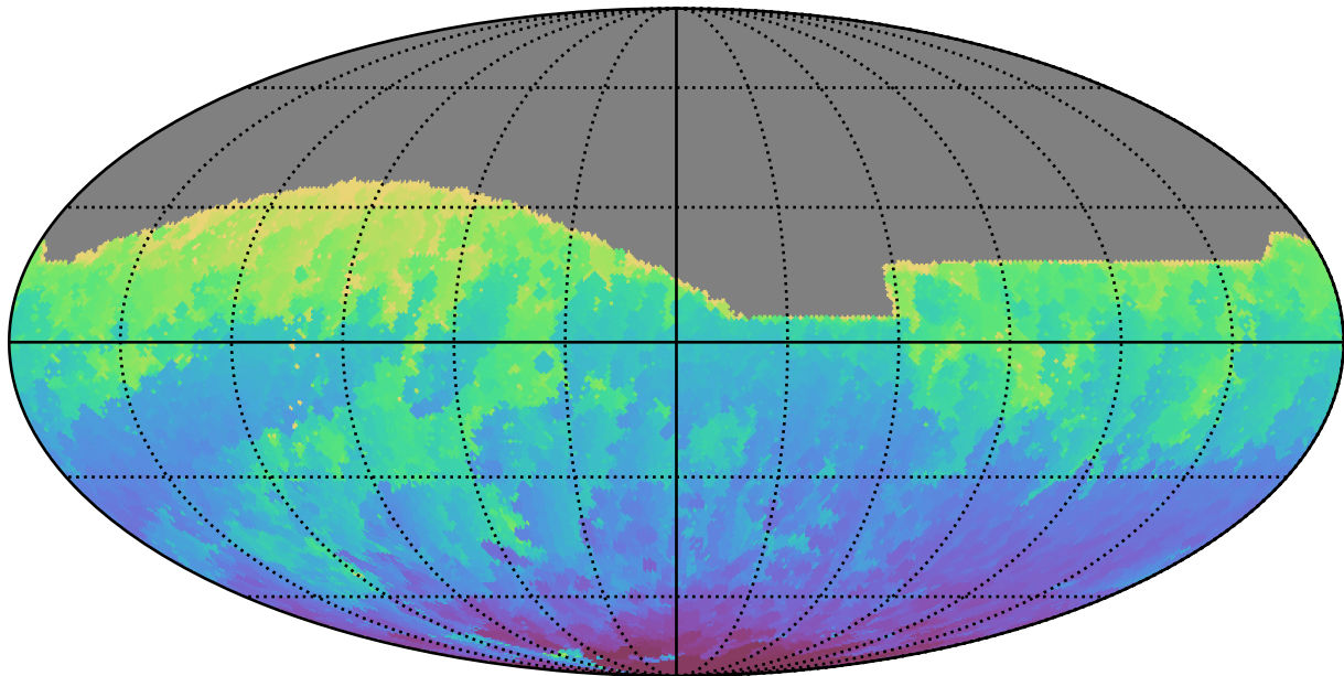
too_100_4v3.4_10yrs All sky i band: Min HA
