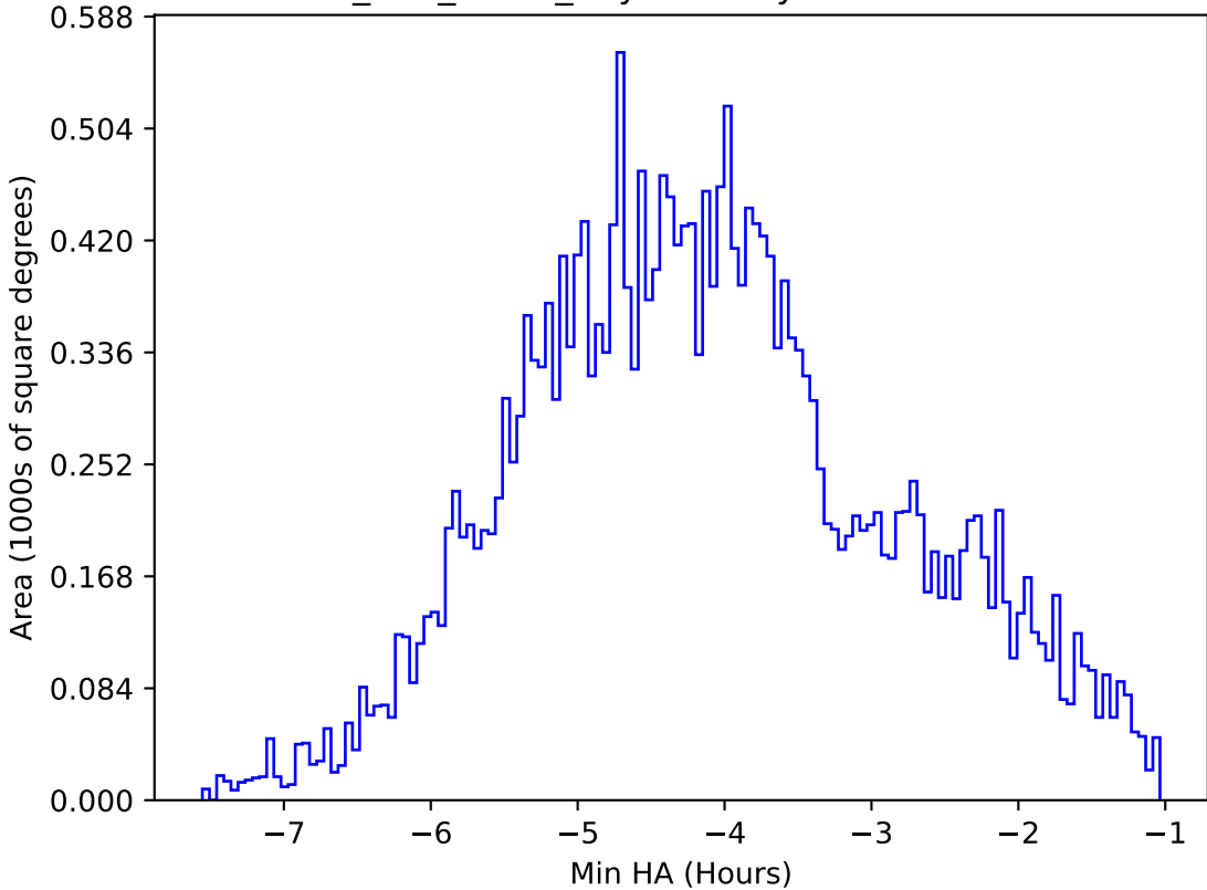
too_100_4v3.4_10yrs All sky i band: Min HA
