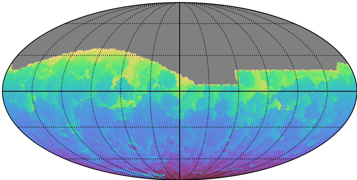
too_100_4v3.4_10yrs All sky g band: Min HA
